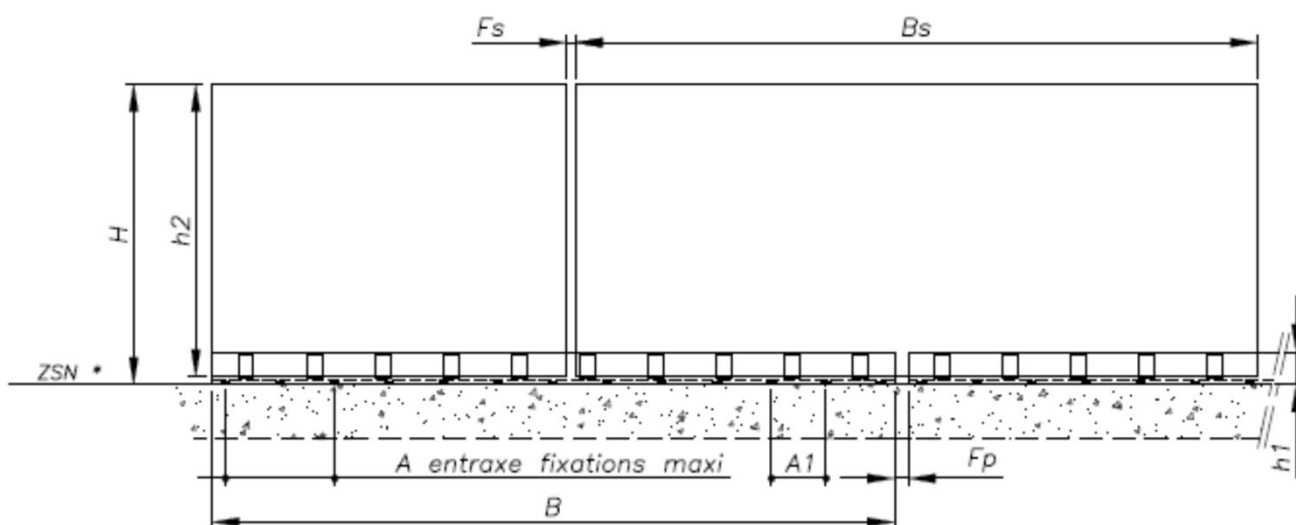
Figure 16 – Pose sur dalle – Modèle SW - 8050
