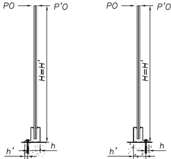
Figure 14 – Dimensionnement des chevilles de fixation pour le cas du système 7017 / 7017R / 7018L
